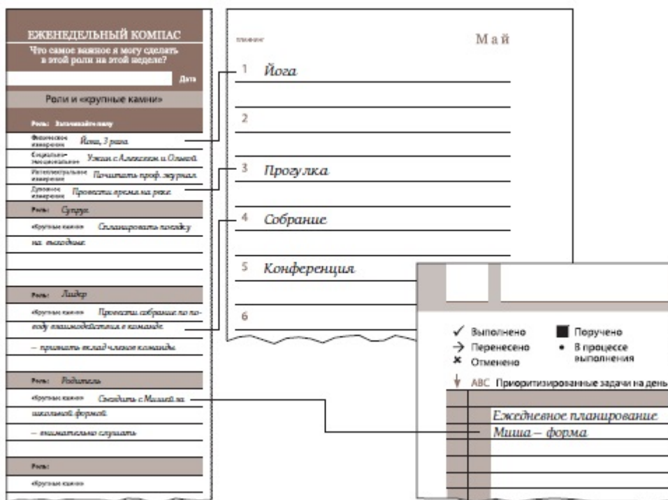
Рис. 4. Ежедневное планирование
